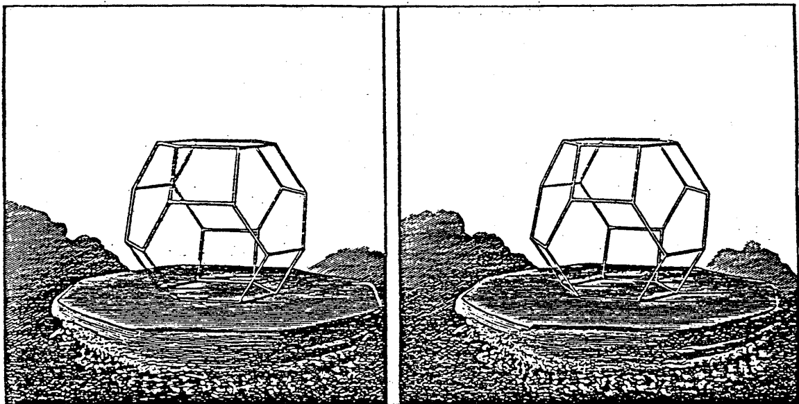
第2図 Kelvin の14面体の立体図：4角形面6ケと6角形面8ケをもつので(0608)と分類される。
