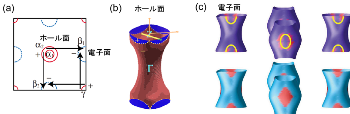
図 2 : (a) 鉄系超伝導体のホールのフェルミ面と電子のフェルミ面 (2 次元面内) [4]. 色の違いは超伝導秩序パラメータ \Delta の符号の反転を表している (s±波超伝導). (b) ホール面の Z 点付近の水平ノード [10]. (c) 電子面上のループ状ノード [12].
