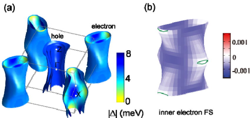
図7 : \text{BaFe}_2(\text{As}_{1-x}\text{P}_x)_2 の超伝導ギャップサイズ |\Delta| (a) ARPESにより観測された |\Delta| の運動量分布. (b) スピン揺らぎと軌道揺らぎを考慮した理論により計算された内側電子面の超伝導ギャップ異方性[23]. 緑線はノードを表している。
