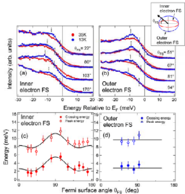
図6 : \text{BaFe}(\text{As}_{1-x}\text{P}_x)_2 ( x=0.30 , T_c=30\text{K} )の2枚の電子面における超伝導ギャップの異方性 ( \hbar\nu=40\text{eV} ). (a)(b) T_c 以上( T=35\text{K} )及び T_c 以下( T=13\text{K} )で観測されたEDC. (c)(d) EDCのピークエネルギーおよび T_c 上下のスペクトルの交点のエネルギー。超伝導ギャップの大きさを反映している。
