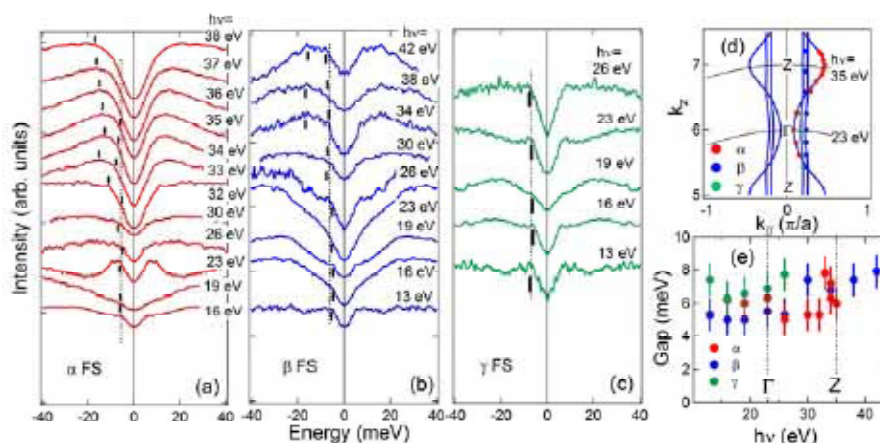
図5 : \text{BaFe}(\text{As}_{1-x}\text{P}_x)_2 ( x=0.30 , T_c=30\text{K} )の3枚のホール面における超伝導ギャップの k_z 依存性。(a)-(c)フェルミ面上の対称化された EDC。(d) 運動量空間における測定点。(e) 超伝導ギャップの励起エネルギー依存性。
