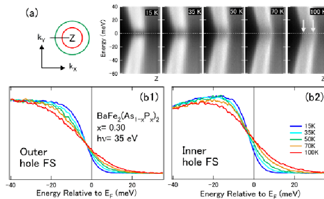
図4 : \text{BaFe}(\text{As}_{1-x}\text{P}_x)_2 ( x=0.30 , T_c=30\text{K} )のホール面Z点付近の超伝導ギャップ。(a) 左図のカットに対応する対称化された ARPES スペクトルの温度変化。(b1)(b2)外側および内側のフェルミ面上のエネルギー分布曲線(EDC)
