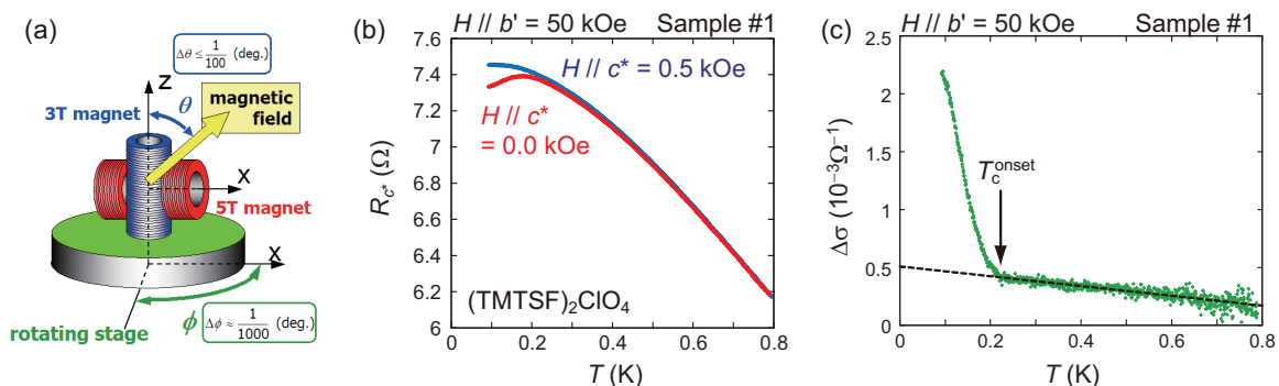
図 4: (a)本研究で用いた磁場方向制御装置ベクトルマグネット[22]. 二つの超伝導マグネットと回転台を組み合わせ、3 次元的な磁場方向の精密制御を可能にした. (b) T_c^{onset} 決定のためのデータの例. 磁場を導電面 ( ab' 面) に並行にかけた場合 (赤いグラフ) と、更に c^* 軸方向に微小な磁場を加えた場合 (青いグラフ) の電気抵抗の温度依存性を比較すると、低温域でのみ大きな差異が見られる. (c) 2 つの電気抵抗から電気伝導の差 \Delta\sigma = R_{c^*}^{-1}(H_{c^*} = 0 \text{ kOe}) - R_{c^*}^{-1}(H_{c^*} = 0.5 \text{ kOe}) をとったもの. 電気伝導 \Delta\sigma の急激な上昇から T_c^{onset} を定義した.
