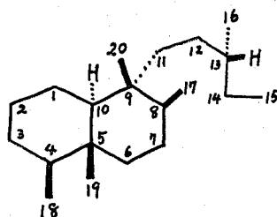
Clerodane
