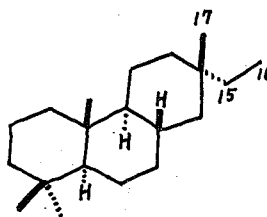
Isopimarane
