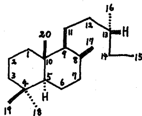
Labdane
