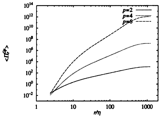
図 16: r/\eta に対する \Pi_r の p 次のモーメント \langle \Pi_r^{G,p} \rangle . p = 2, 4, 6 . R_\lambda = 395 .
