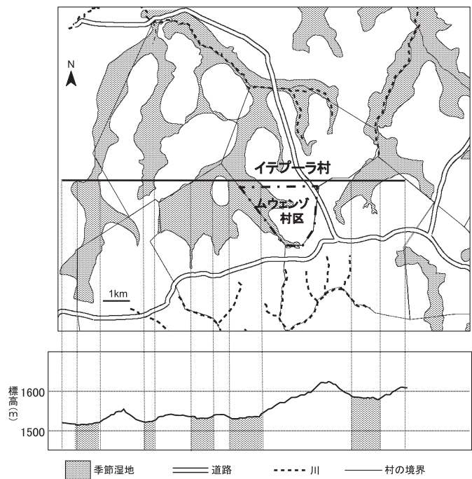
図 2 調査地における季節湿地の分布と標高断面図
