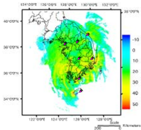
図1 合成されたレーダーコンポジット画像 (2002年8月31日15時)
