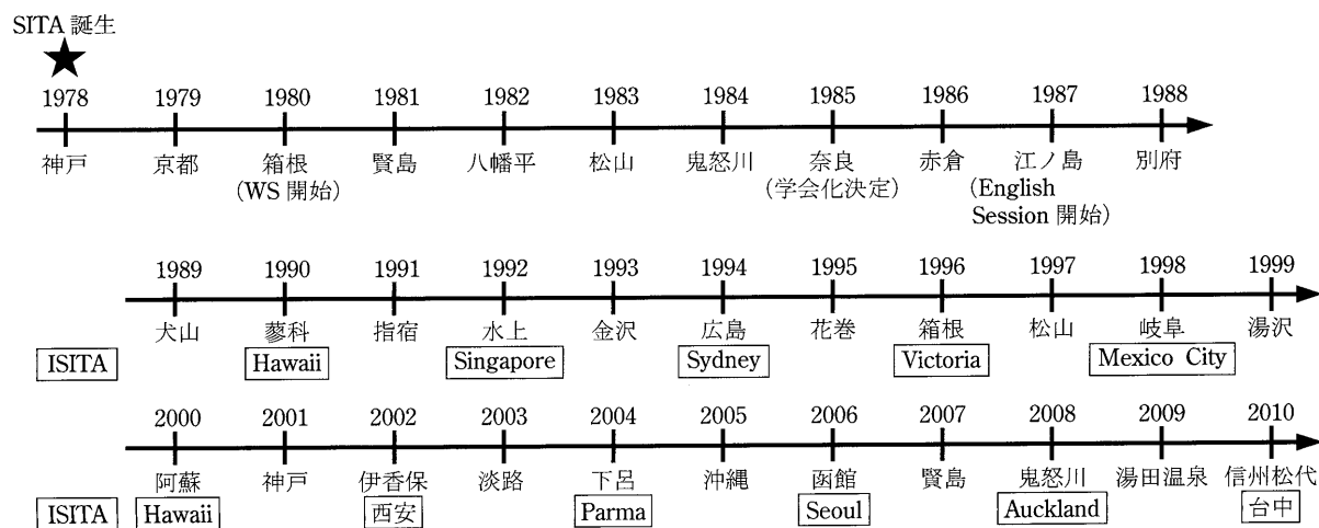
図 1 SITA の歴史
