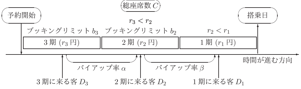
図 2: パイアアップがある 3 期間静的レベニューマネジメントモデル.
