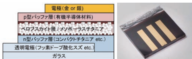
ペロブスカイト型太陽電池
