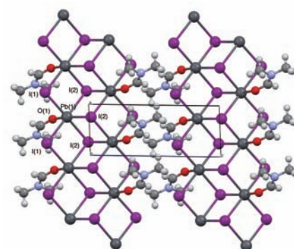
\text{PbI}_2 \cdot \text{DMF} 錯体のX線結晶構造
