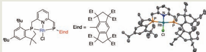
Eind基を導入したPPEPを有するRh錯体
