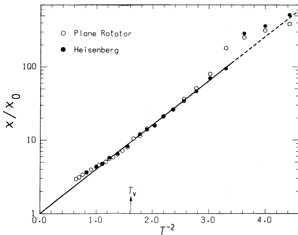
図1 正方格子に配列したハイゼンベルグ・スピン系のモンテカルロ法によって決められた秩序変数の温度依存性。実線は最小自乗法で (1 - T/T_c)^\beta に適合するように決めたものである。
