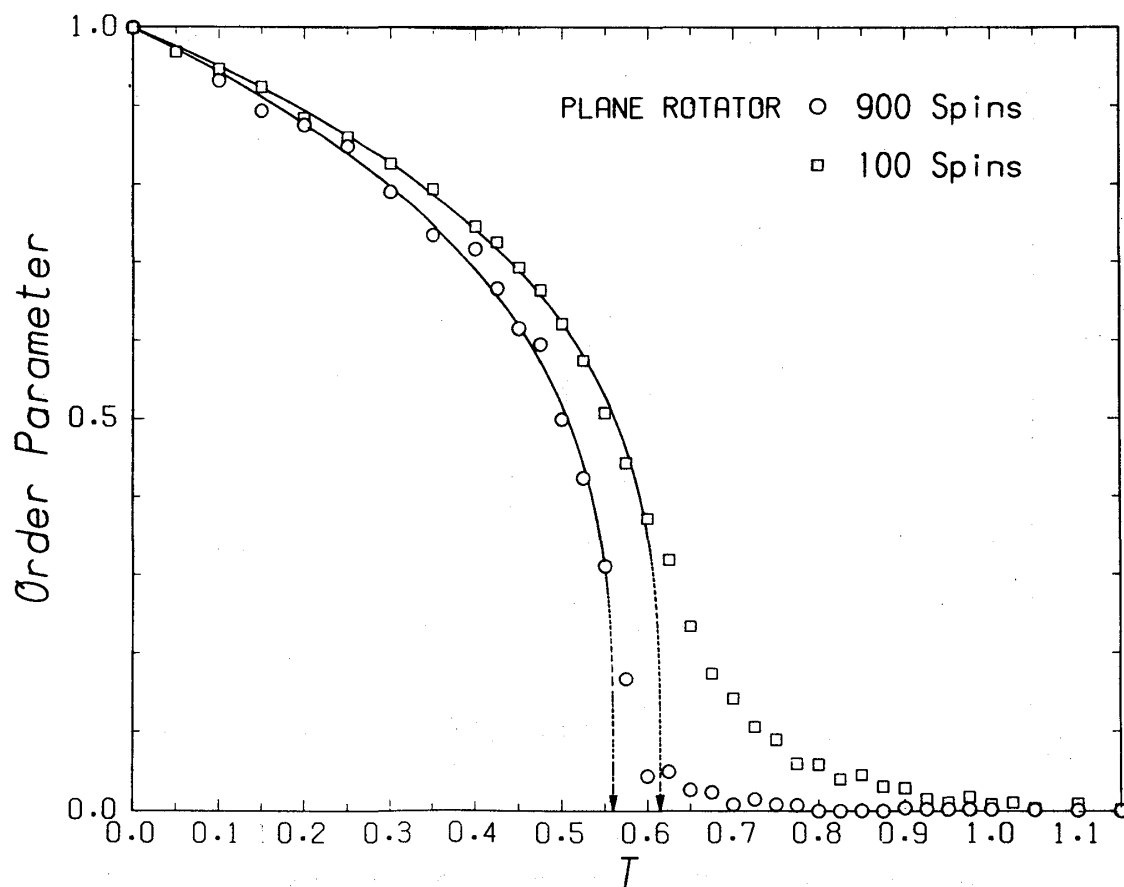
図2 正方格子に配列した平面回転子系のモンテカルロ法によって決められた秩序変数の温度依存性。
