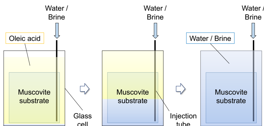
図 1. オレイン酸中の白雲母基板表面の水相による掃攻実験。水相を 100 mM \text{CaCl}_2 水溶液、100 mM \text{NaCl} 水溶液、精製水とし、それぞれに対して同様に掃攻実験を実施。
