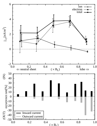
図 1. Geotail 衛星による電流の観測
