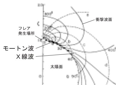
図2. フレアに伴う衝撃波のモデル
