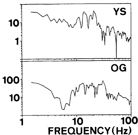
Fig. 6. Power spectra of coda waves. Upper: YS site. Lower: OG site.
