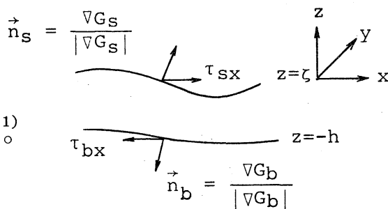
図2 \tau_{sx}, \tau_{bx} の正の向き
