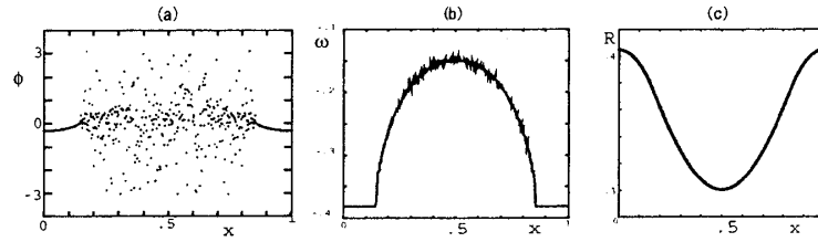
図 5: 非局所結合位相モデル (5.4) から得られた 1 次元のキメラパターン. (a) 個別振動子の位相分布 (スナッピングショット), (b) 個別振動子の振動数分布, (c) オーダーパラメタ R のパターン.
