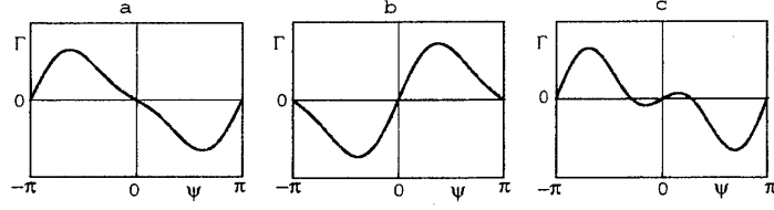
図 2: 位相結合関数の代表的 3 タイプ.
