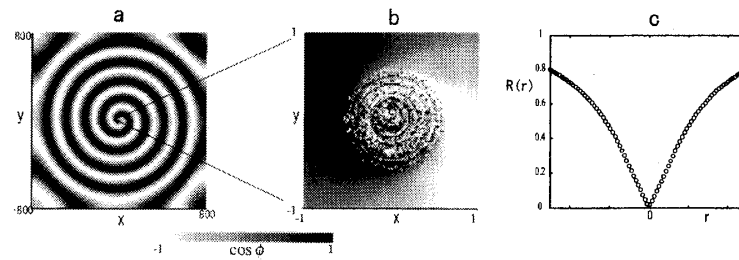
図 6: キメラ構造をもつらせん波パターン. (a) のように全体のパターンは正常ならせん波パターンに似ているが, 中心付近では (b) のように振動子の位相はまったくばらばらになっている. オーダーパラメタの振幅 R の動径方向に沿ってのプロフィールは, (c) のように正常ならせん波と何ら変わらない.
