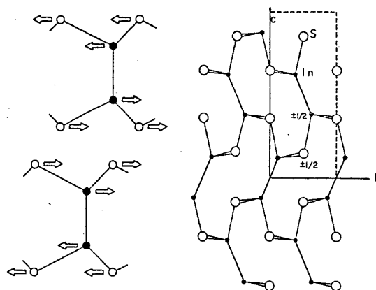
Fig. 4 (a) 55\text{ cm}^{-1} E'' モードの変位ベクトル
