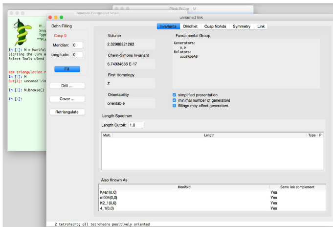
図 6: browse 機能
