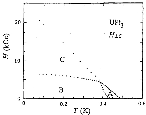
図10 \text{UPt}_3 の多重超伝導相図 (S. Adenwalla et al. )
