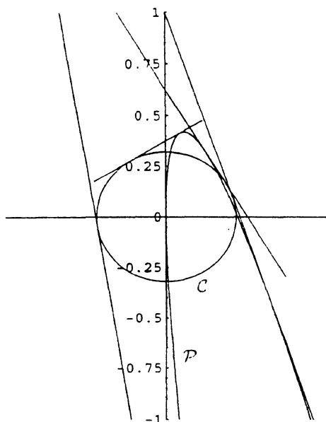
図 2: 4 次方程式の解法例
