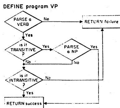
図 4 PROGRAMMAR による文法記述
