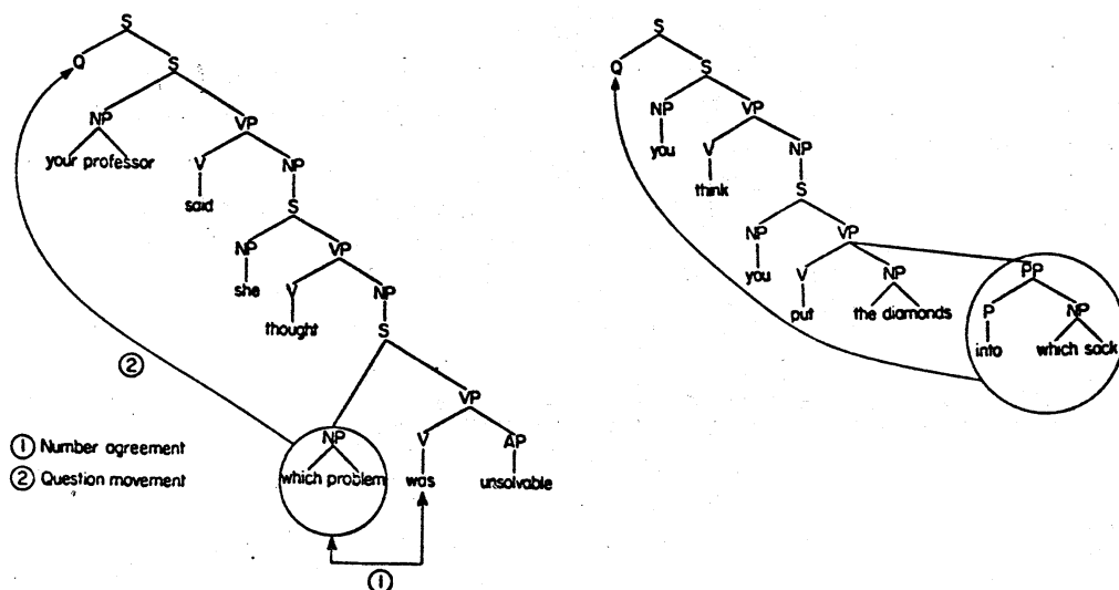
図3 変形規則 — movement 規則の例
