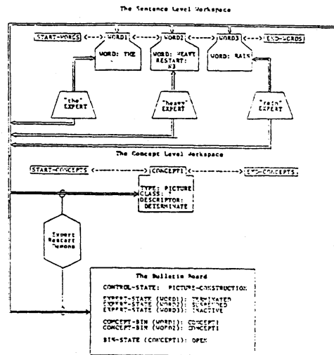
図8 Rieger の Word Expert Parser の概念図
