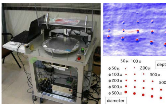
図5：過流探傷装置と疑似欠陥の測定結果
