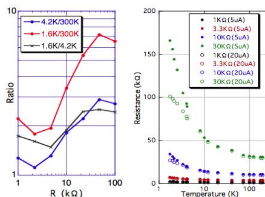
図10：酸化ルテニウム抵抗の温度特性
