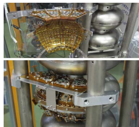
図 1 2 : 試作基板の実装 空洞の 1 セル 45° 部分（基板 4 枚）に試作基板を実装
