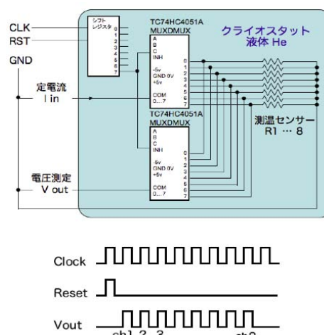
図8：T-map 回路
