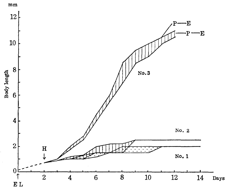
図1 Chironomus sp. の成長曲線 (T. Mizuno, 1973)
