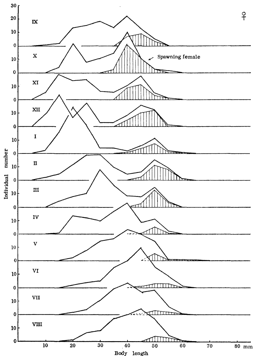
図2 テナガエビの一種 Macrobrachium trompi の雌の体長分布と抱卵個体(T. Mizuno, 1974)
