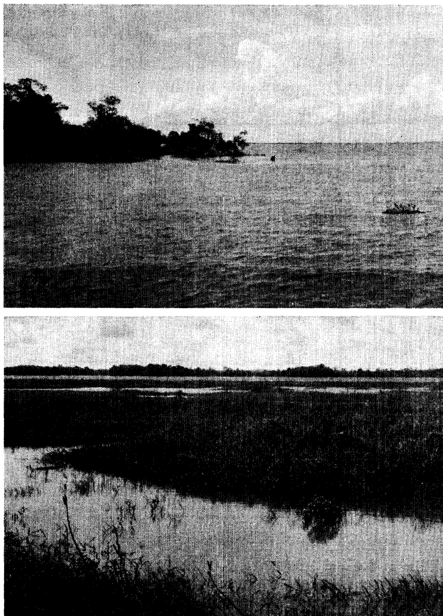
図3 東カリマンタン，Mahakam 河水系における湿原湖沼の景觀 （上）開水面は広大であるが，深度は2-3mで浅い。 （下）周辺部は水草群落や浮島が発達している。
