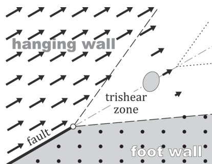
Fig. 18. Schematic cross-section illustrating the trishear fault-propagation model. The gray ellipse represents the strain in the trishear zone. 断層伝播褶曲のモデル。トライシアーを説明するための模式的断面図。灰色の楕円は、trishear zone のなかの歪み楕円を模式的に示す。
