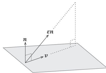
Fig. 3. Shear strain acting on the plane with the unit normal, \mathbf{n} , has the maximum along the direction, \mathbf{v} , that is the orthogonal projection of \boldsymbol{\varepsilon} \mathbf{n} onto the plane. 単位ベクトル \mathbf{n} に直交する面に作用する剪断歪みは、 \boldsymbol{\varepsilon} \mathbf{n} をその面に正射影した方向 \mathbf{v} で最大になる。
