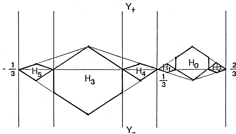
Fig.3.4.4. Hexagones H_0 , H_3 and quadrilaterals H_1 , H_2 , H_4 , H_5 .
