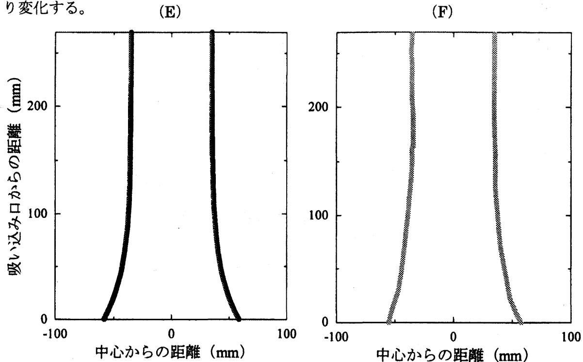
Fig.9 渦糸対の形状 (数値計算の結果と実際の形状)
