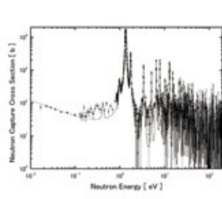
原子炉実験所の電子線型加速器で測定したアメリシウム243の中性子捕獲反応断面積
