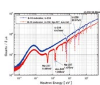
非破壊分析のために測定した透過中性子スペクトルの一例
