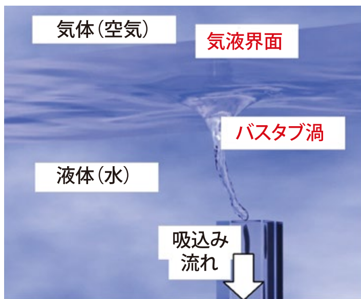
バスタブ渦の解析結果
