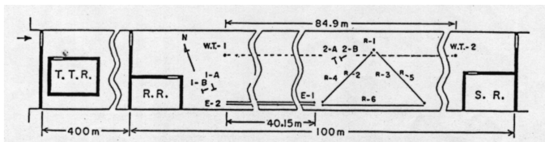
Fig.2 計器配置図
