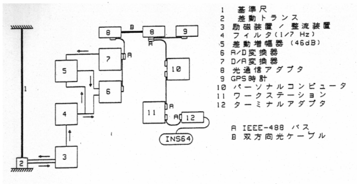
ブロック図
