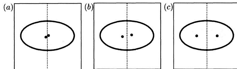
図 9: 細胞形状は楕円形であり ( a = 4.0 \times 10^{-5} , b = 2.3 \times 10^{-5} )、化学物質は存在しない ( \kappa_r(t) \equiv 0 , \kappa_a(t) \equiv 0 ): (a) は初期状態、(b) は途中経過、(c) は最終状態。
