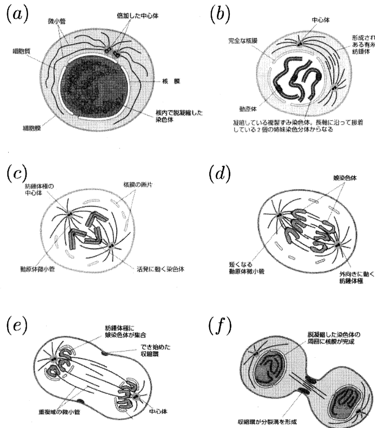
図 2: 細胞分裂の過程. (a) は間期、(b)~(f) は M 期の様子である. [8] より転載.
