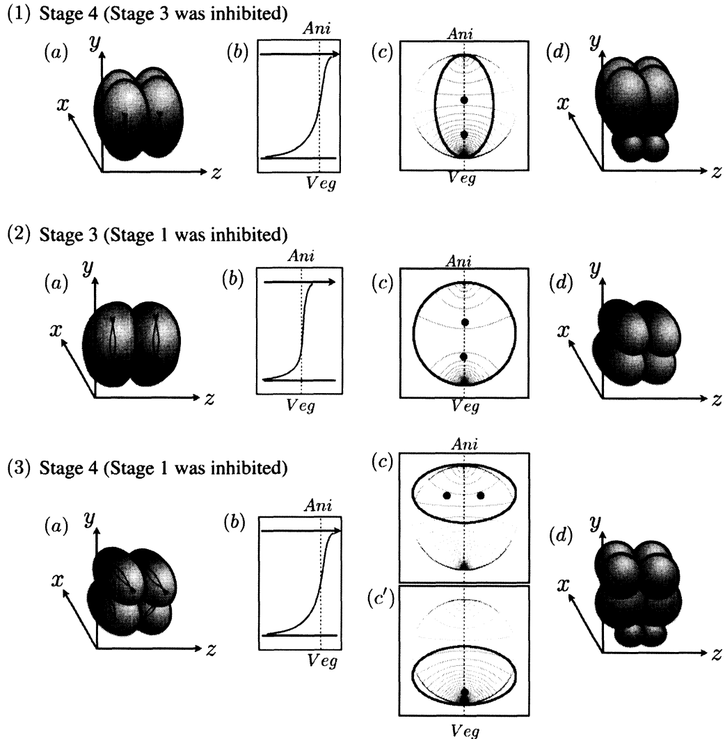
図 13: 卵割の阻害実験の数値計算結果. (1) では第 3 卵割が, (2), (3) では第 1 卵割が阻害された実験である. パネル (a) は実験での卵割直前の概略図. パネル (d) は実験での卵割直後の概略図. パネル (b) は AV 軸に沿う \psi のプロファイルを表す. パネル (c) はシミュレーションの最終状態を表す. それぞれのパネルにおいて y 軸は AV 軸と平行になるようにとられている. (1) Stage 4: t = 120 , (g_x, g_y) = (0, 0) , a = 2.3 \times 10^{-5} , b = 4.0 \times 10^{-5} (2) Stage 3: t = 90 , (g_x, g_y) = (0, 0) , a = b = 4.0 \times 10^{-5} (3) Stage 4: t = 120 , (g_x, g_y) = (0, \pm 1.88 \times 10^{-5}) , a = 4.0 \times 10^{-5} , b = 2.3 \times 10^{-5}
