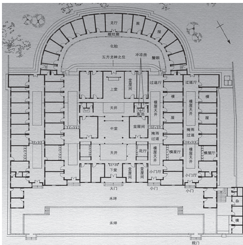
前掲「東華廬平面図」『梅県三村』106頁
