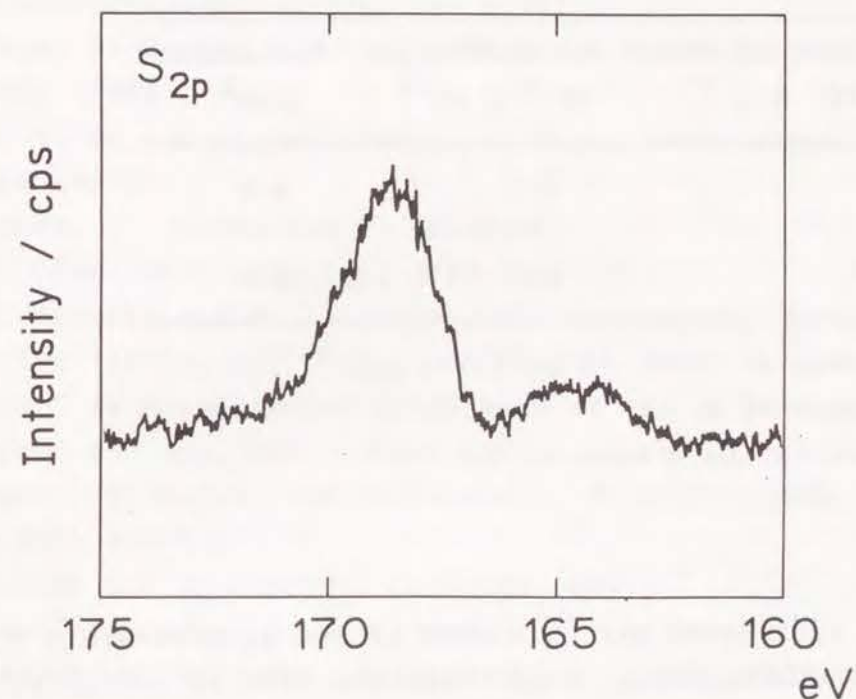
Fig. 3.11. ESCA \text{S}_{2\text{p}} spectrum of plasma polymer of Fig. 3.10.
