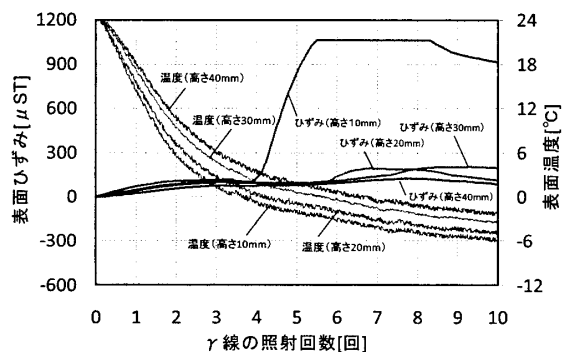
図 4 気泡無し ALC の表面ひずみおよび表面温度（凍結過程）
