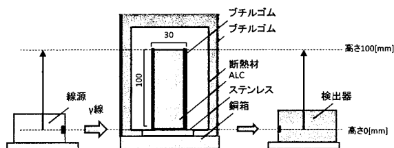
図2 実験装置の模式図
