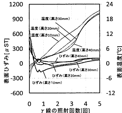
図 8 気泡有り ALC の表面ひずみおよび表面温度（融解過程）
