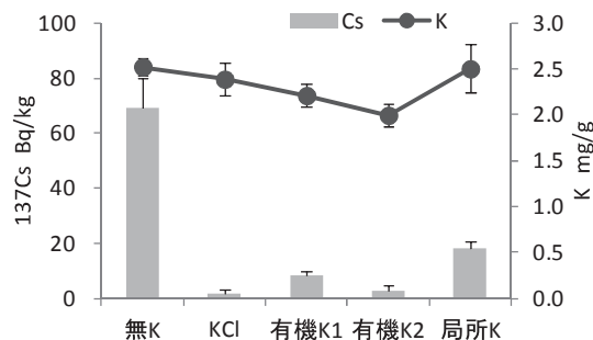
図2 各カリウム肥料施肥によるダイズの放射性セシウム濃度
