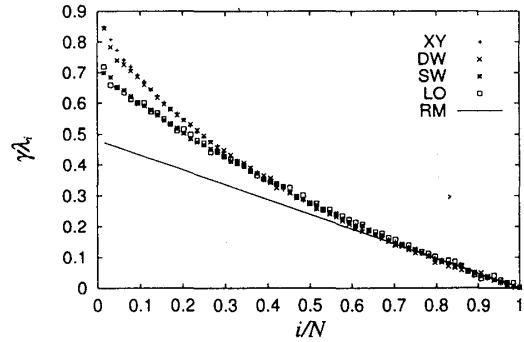
図 1: カオスが Stochastic ほど強くない系におけるリアプノフスペクトルの普遍性。自由度 N = 4^3 = 64 。領域 i/N > 0.4 では系によらない同じ形が得られる。直線は、発達したカオス系で得られる直線スペクトルを示している。
