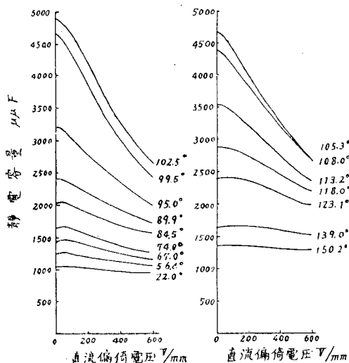
第3圖 温度とパラメーターとした \text{BaTiO}_3 静電容量の直流偏倚電圧特性 428\text{ V/mm} 600\text{ } \mu\text{F}
