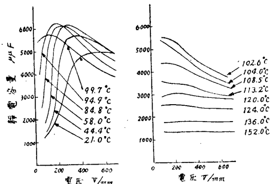
第1圖 溫度をパラメーターとした \text{BaTiO}_3 靜電容量の電圧特性 測定周波数 60\text{C/s}
