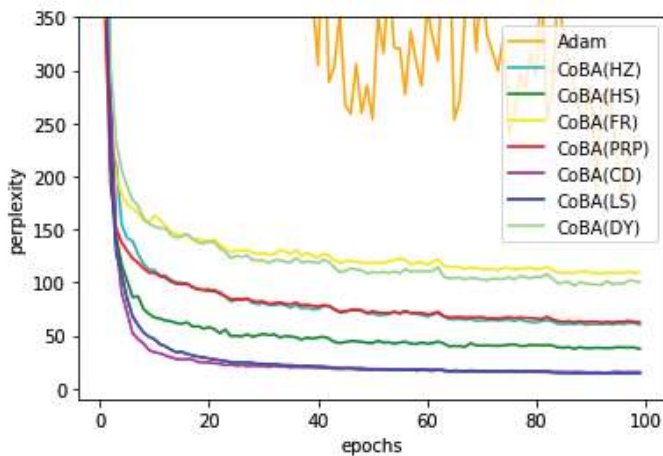
図 1: 既存手法と提案手法それぞれの各エポックにおけるパープレキシティ
