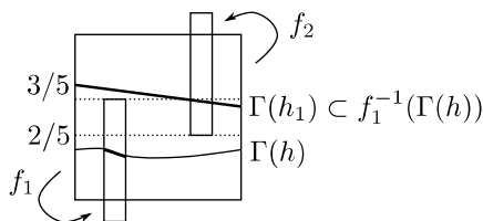
図 1 反復関数系 F = (f_1, f_2)
