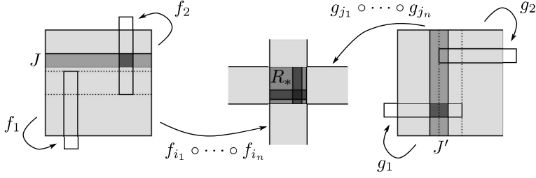
図2 定理 5.2 の証明
