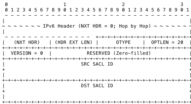
図3 SACL ID を付加するためのパケットフォーマット
