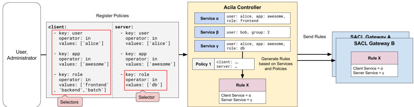
図5 ポリシーの管理と配布
