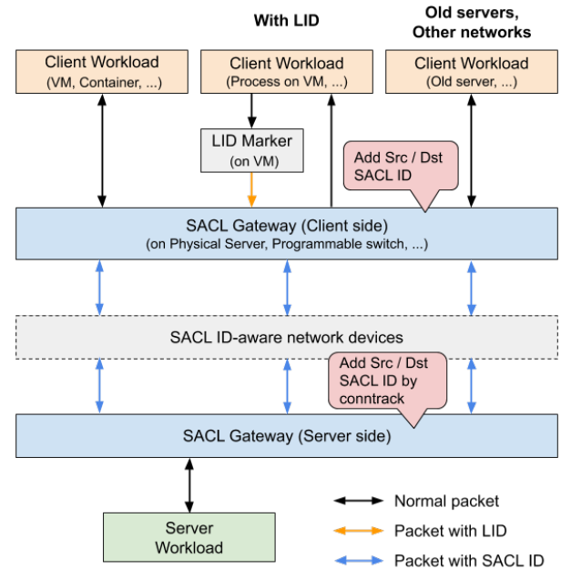
図4 パケットへの SACL ID の付加
