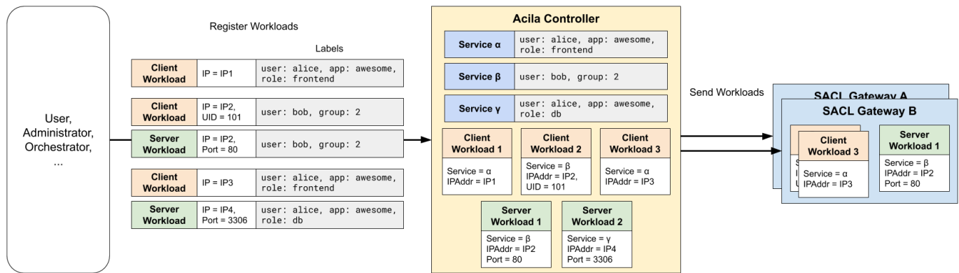
図2 Workload への Service の付与と SACL Gateway への配布
