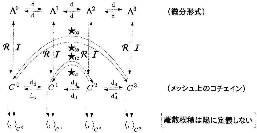
図 1: 提案する離散化の枠組み.
