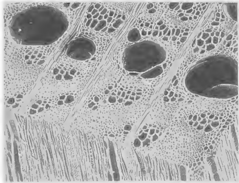
写真10-38 ケヤキ材の走査電顕像
