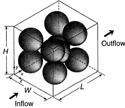
図 2.2 3次元多孔質構造モデル.
