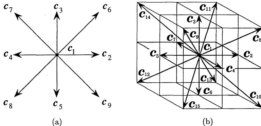
図 2.1 格子気体モデル：(a) 2 次元 9 速度モデル，(b) 3 次元 15 速度モデル。
