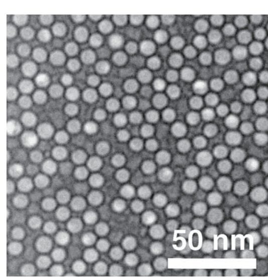
ナノ粒子
