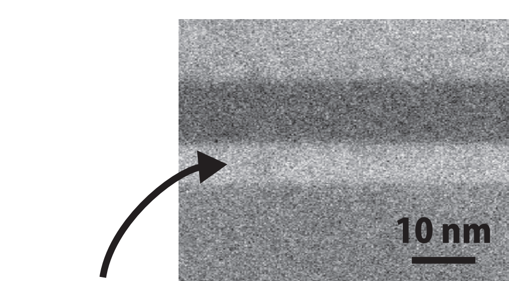
量子井戸
