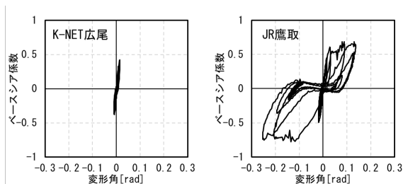
図4 ベースシア係数と変形角の関係
