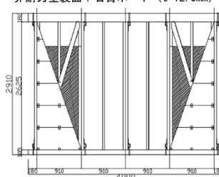
図1 試験体立面図 (WL-BR)
