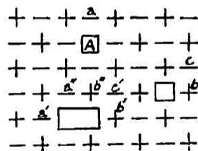
第二十一圖 アルカリイオン、 ハロゲンイオンの 穴及び、"Assozi- ierte Löcherpaar"
