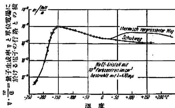
第十二圖 NaCl-結晶に於ける電子行路に對する温度の影響
