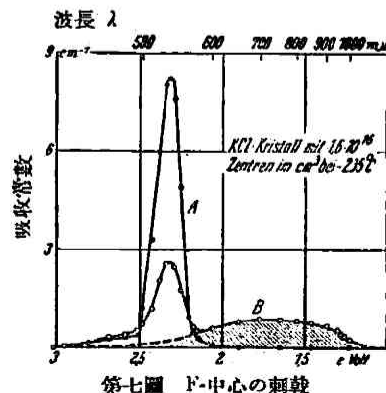
第七圖 F-中心の刺激
