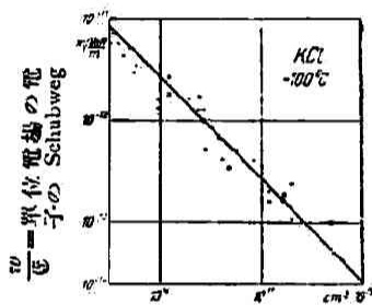
第十四圖 單位電場に於ける Schubweg と F-中心の濃度との關係
