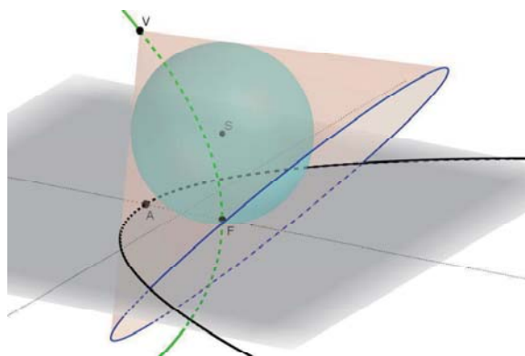
図 7: 放物線の自己双対性.
