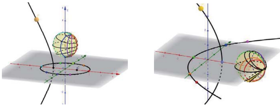
図 9: 楕円を双曲線の 1 つの枝から見た場合 (左) と、放物線を放物線から見た場合 (右).
