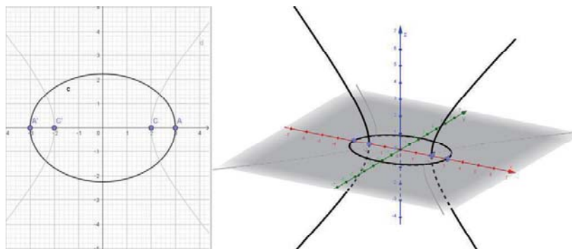
図 5: focal conics の作図.
