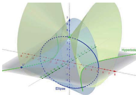
図 6: focal conics の双対性.
