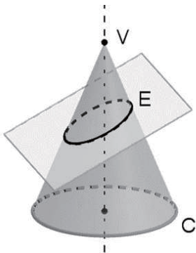
図 1: 「エレガントな解答をもとむ」に掲載された図.
