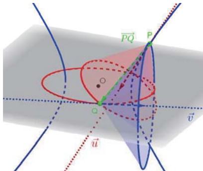
図 10: 直交する2つの円錐.
