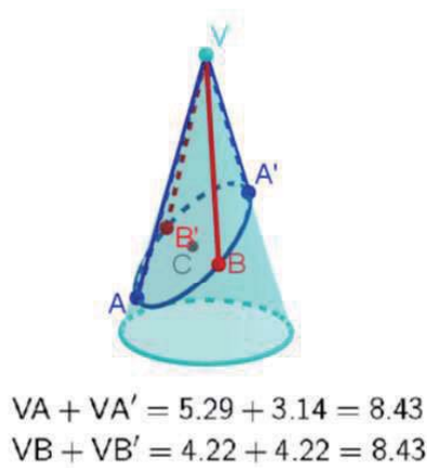
図 3: 円錐の頂点からの距離の和。
