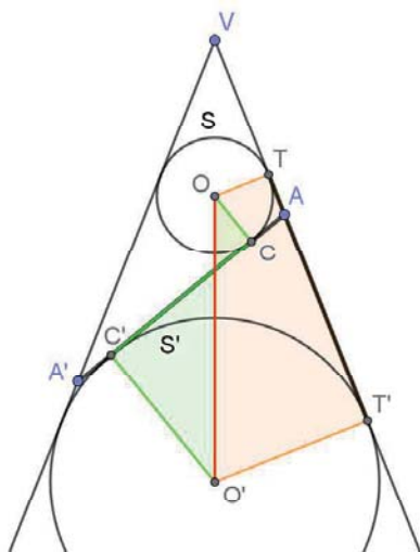
図 4: 2つの Dandeline 球の半径と中心間の距離。
