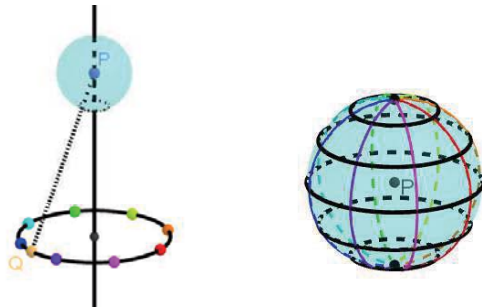
図 8: 円をその軸から見ることによって得られる球面図形.
