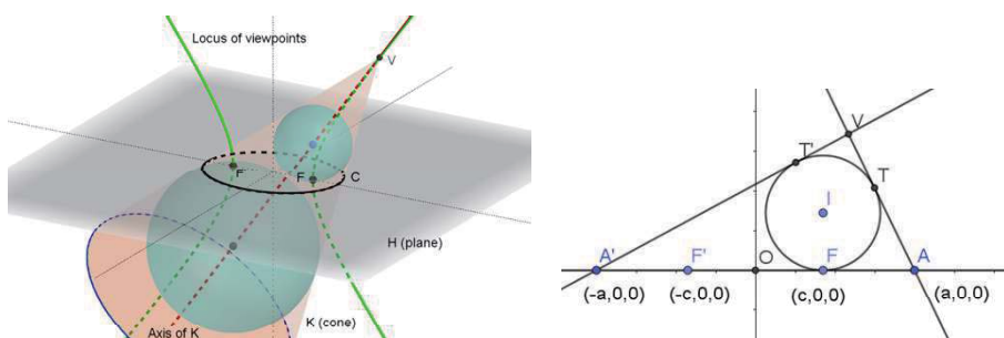
図 2: Dandeline 球 (左) とその断面 (右).
