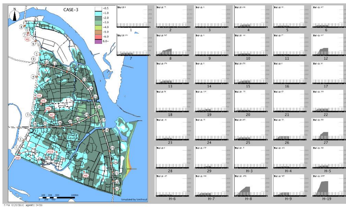
図 44 ケース 3： 1214 秒後（避難終了）
