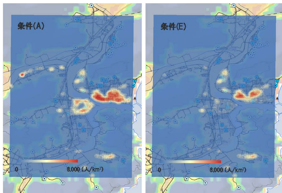
図 8 避難完了時間が 5 分以上となる住民の分布
