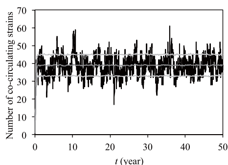
図 3. 同時流行株数の時間発展
