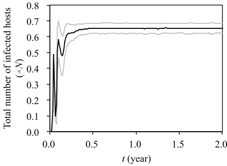
図 1. 総感染者数の時間発展
