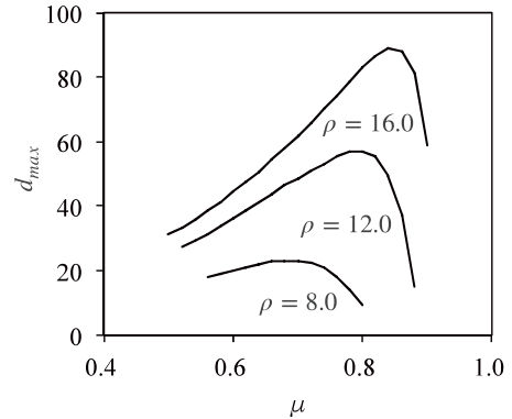
図 2. 最大抗原距離
