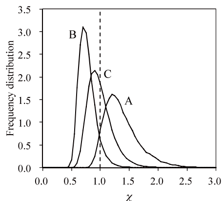
図 4. 単一株の変異株産生能力の分布
