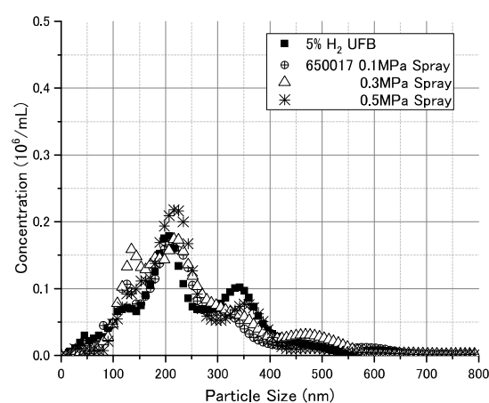
Fig. 3 UFB distribution (Upper: O 2 UFB, Lower: 5%H 2 UFB).
