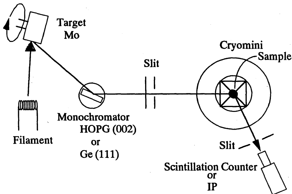
図3.1 光学系
