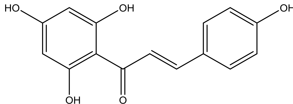
ナリンゲニルカルコンの化学構造
